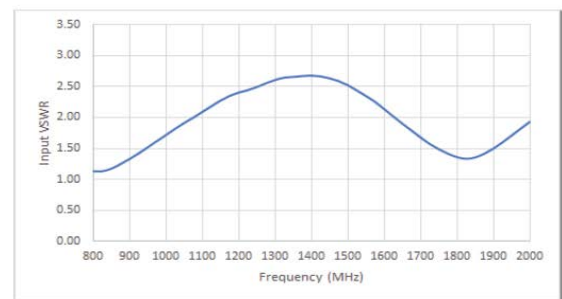
Input VSWR
